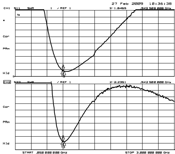
VSWR
