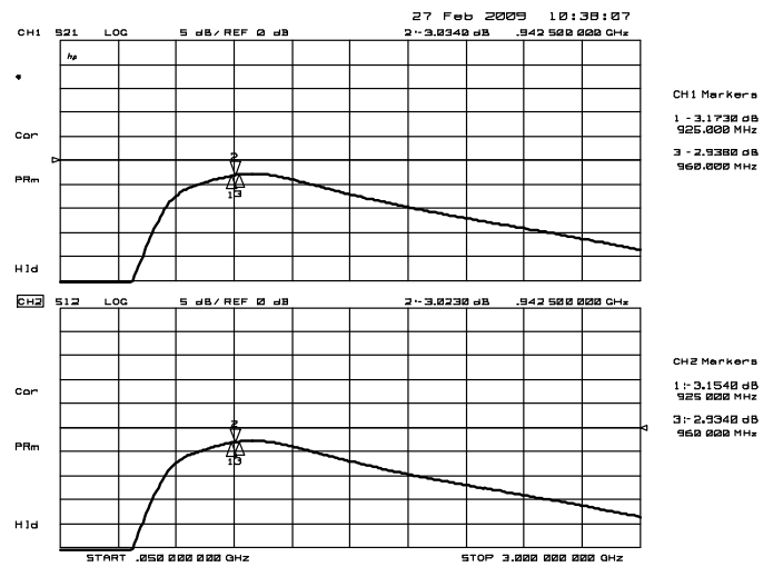
S21, S12
