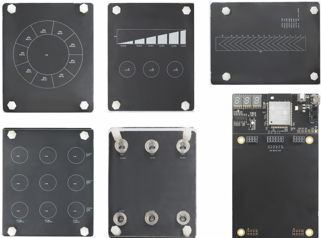
Fig. 1: ESP32-Sense-Kit
