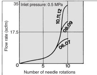
AS3002F
