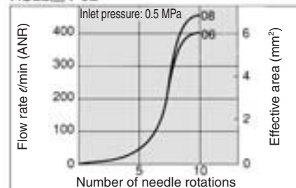
AS22□1-02
