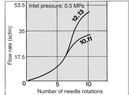
AS4002F
