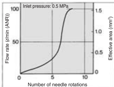
AS1001FG
